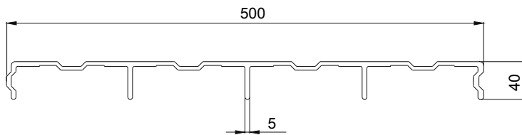
Seitenansicht
