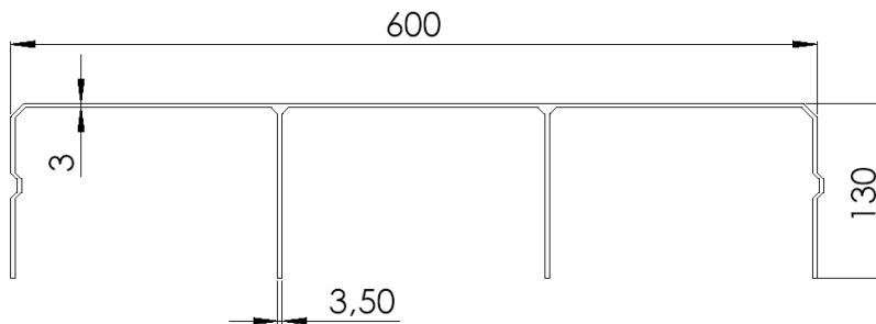
Seitenansicht
